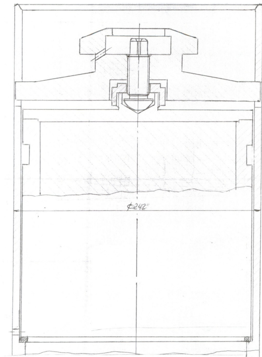
Рис.1 Верхняя часть чехла 24
